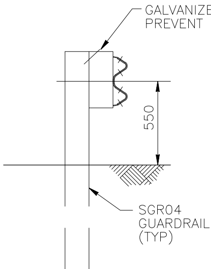
SECTION A-A
